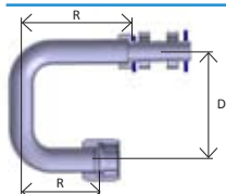
Pag. 17 - "O" ring female swivel - 180°
