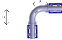
Pag. 21 - 90° elbow splicer
