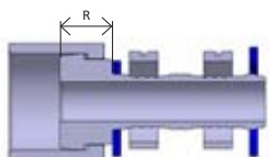
Pag. 18 - ORFS female swivel
