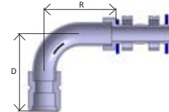
Pag. 15 - 90° elbow
