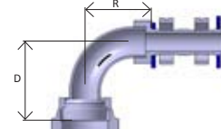
Pag. 18 - 90° elbow
