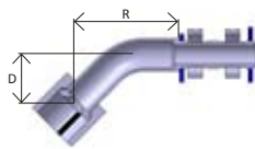
Pag. 5 - 45° elbow
