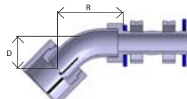
Pag. 18 - 45° elbow
