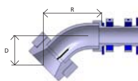
Pag. 19 - "Bock" flange 45° elbow
