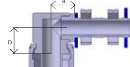
Pag. 12 - 90° elbow
