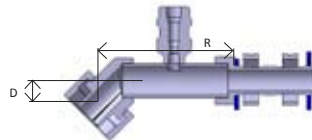
Pag. 9 - 45° elbow
