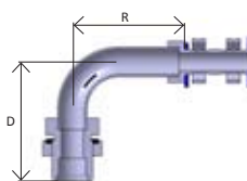
Pag. 17 - 45° elbow
