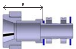
Pag. 19 - "Bock" flange connection
