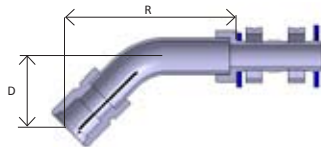
Pag. 15 - 45° elbow
